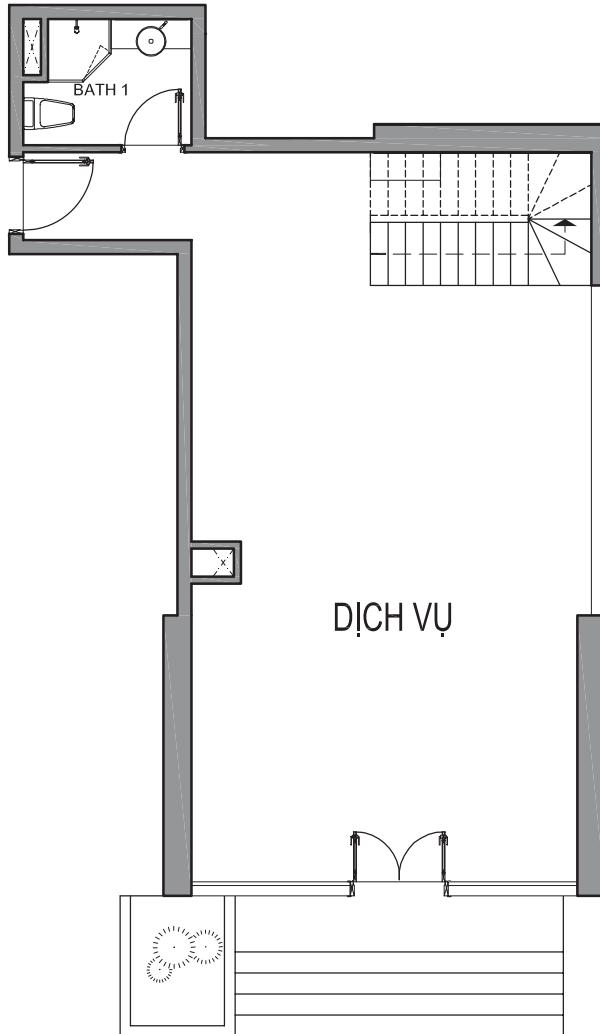
MẶT BẰNG TẦNG TRỆT
